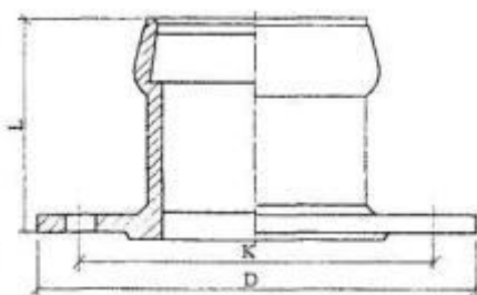
Рисунок 4 - Фланец - раструб E - KS
