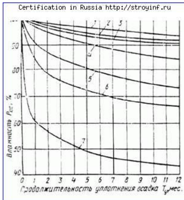
Рис. 3. Средние значения влажности осадка станций осветления и обесцвечивания воды при уплотнении до одного года
