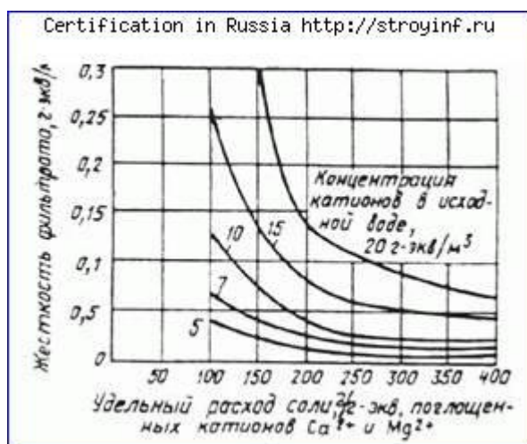
Рис. 1. График для определения остаточной жесткости воды, умягченной одноступенчатым натрий-катионированием
