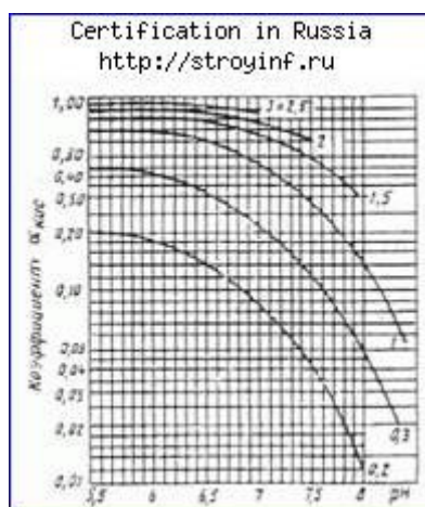
Рис. 3 Номограмма для определения коэффициента \alpha_{кис} при расчете дозы кислоты
