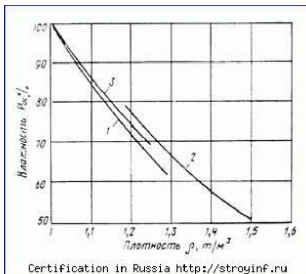
Рис. 6. Значения плотности в зависимости от влажности осадка станции обезжелезивания и реагентного умягчения воды
