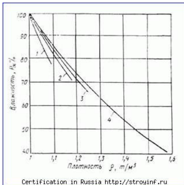
Рис. 5. Значения плотности в зависимости от влажности осадка станции осветления и обесцвечивания воды
