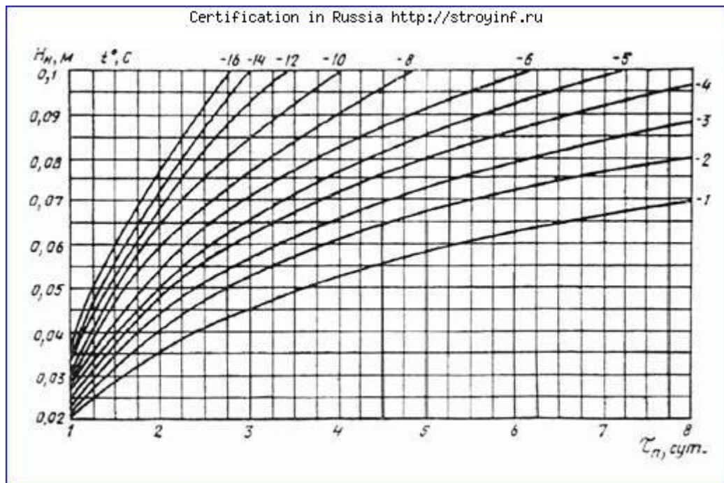
Рис. 7. Зависимость глубины промораживания слоя осадка от среднесуточной температуры воздуха и продолжительности промораживания
