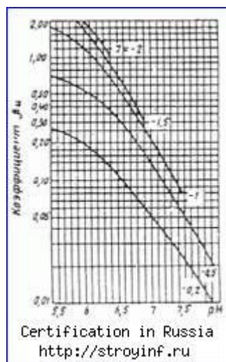
Рис. 4. Номограмма для определения коэффициента \beta_{\text{н}} при расчете дозы щелочи
