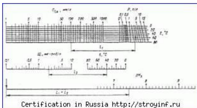
Рис. 1. Номограмма для определения pH насыщения воды карбонатом кальция (pH s )
