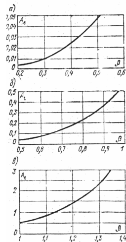
Рис. 2. Зависимость коэффициента \beta от параметра A_t
