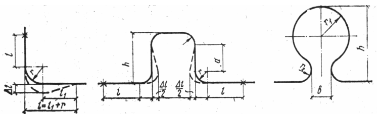
Рис. 3. Основные геометрические параметры
